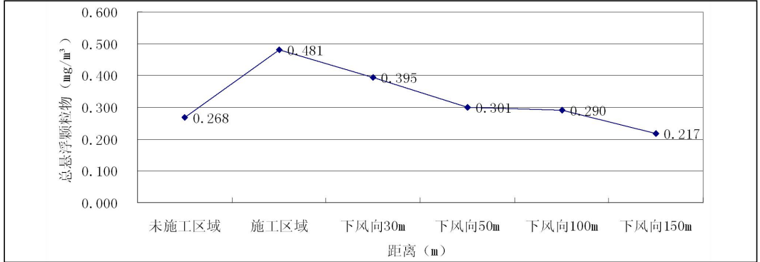
图 7-1 建筑扬尘浓度随距离变化曲线图
